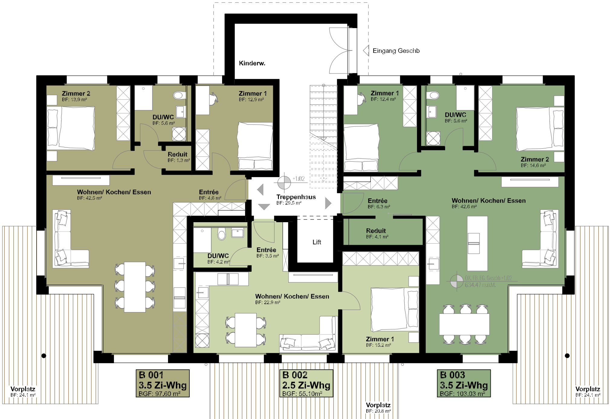
Grundriss Erdgeschoss Geschb Haus B Mst. 1:100
