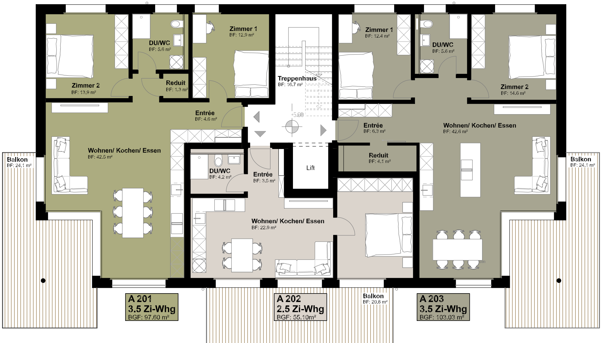
Grundriss 2. Obergeschoss Gescha Haus A Mst. 1:100
