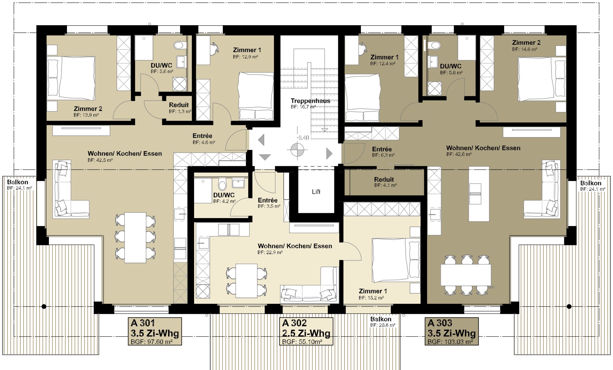
Grundriss Dachgeschoss Gescha Haus A Mst. 1:100
